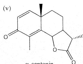
\alpha -santonin
