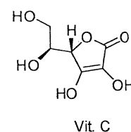
Vit C
