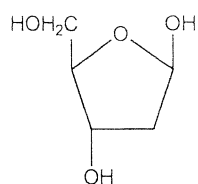
\beta -Deoxyribose
