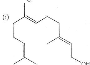
farnesol
